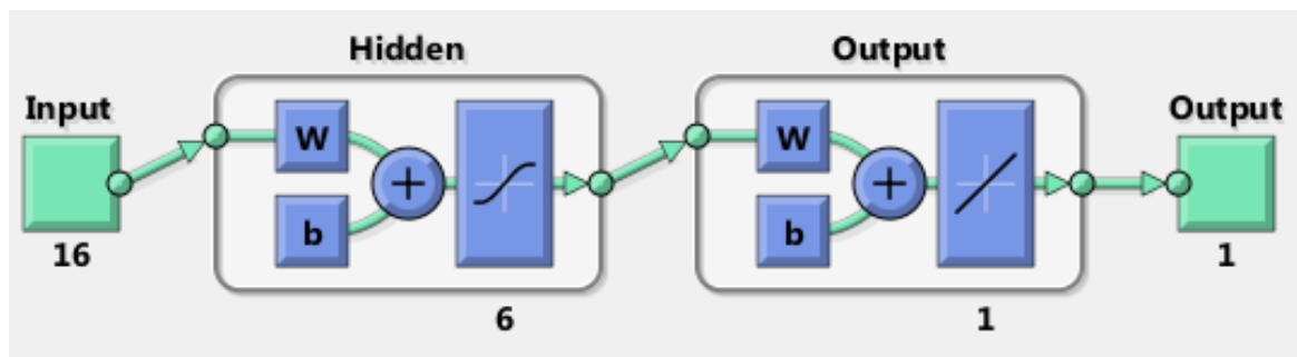
شکل ۲- شبکه عصبی پیش‌رو با ۱۶ ورودی.
