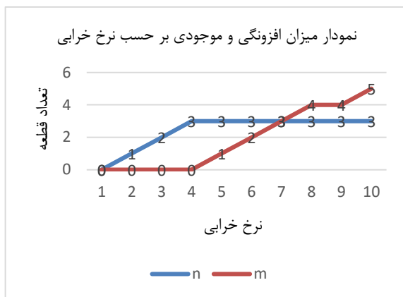
شکل (۲): نمودار میزان افزونگی و موجودی بر حسب نرخ خرابی
